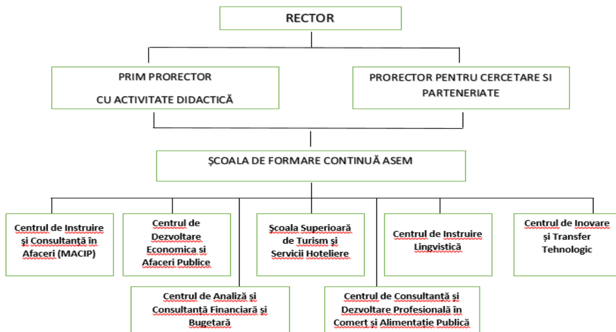
Figura 1. Organigrama SFC
