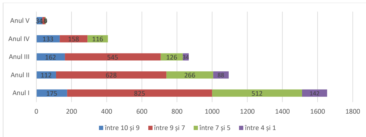
Figura 12 . Structura notelor
